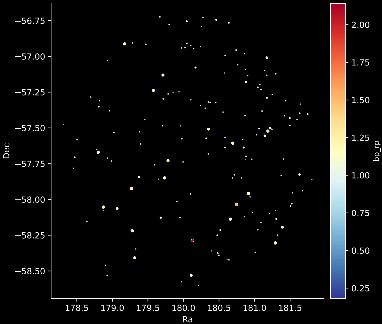
GALAH DR4 Field: [7184] Stars: 151
