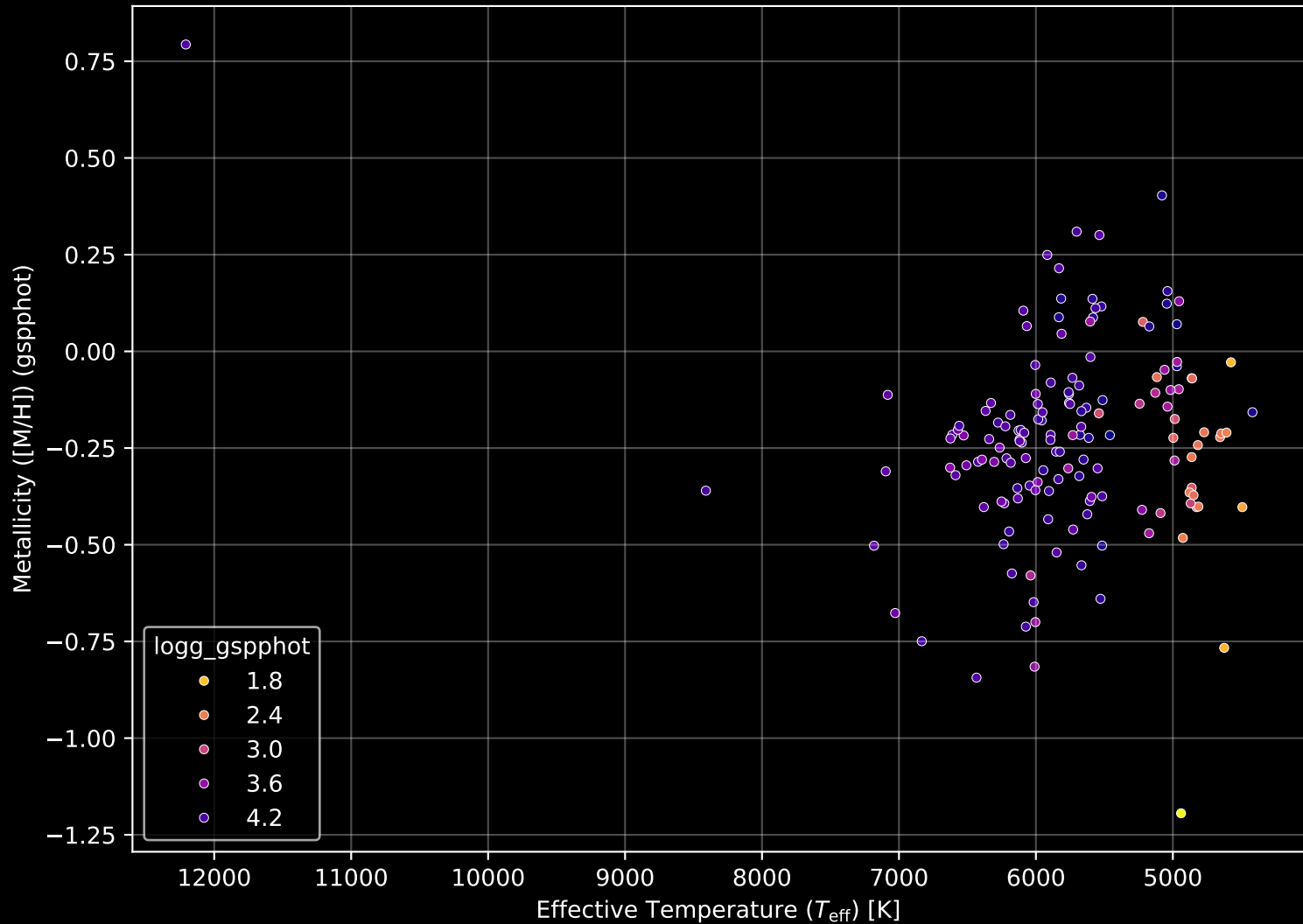
GALAH DR4 Field: [7184] Stellar Population Parameters (n= 151)
